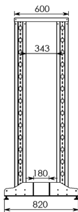
Вид сбоку
