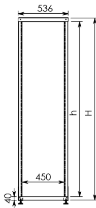
Вид спереди
