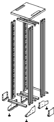
Покомпонентное изображение
