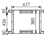
Вид сверху
